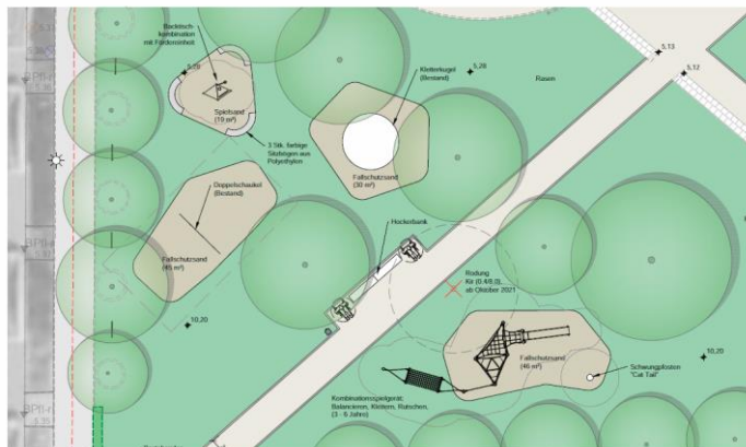
Lageplan Ausschnitt „Spielinseln“
